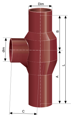
Spiralgrenrør 88°
