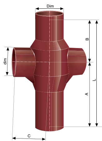
Spiralgrenrør dobbel 88°
