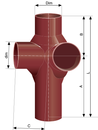
Spiralhjørnegrenrør 88°
