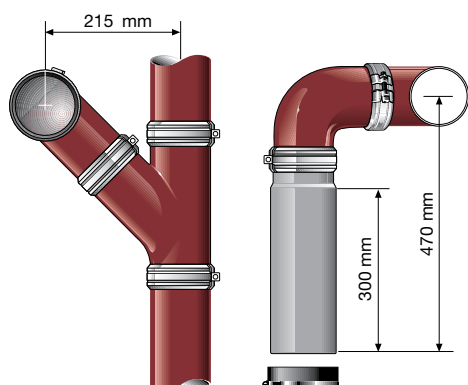
Fig. 4. Tilkobling av klosett til side for vertikal samleledning med 88° bend, 45° grnør og rett, klosett tilkobling, kan kappes.
