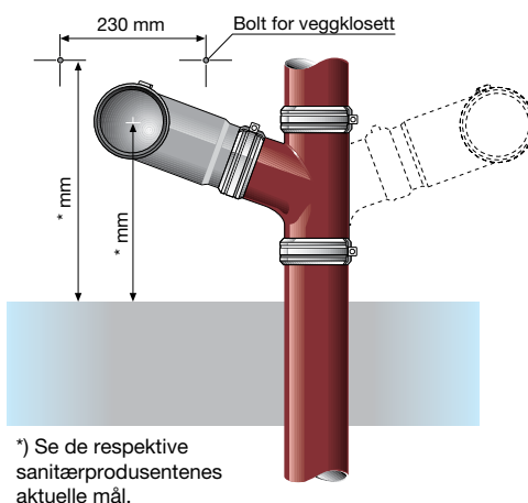
Fig. 3. Tilkobling av ett eller to vegghengte klosetter til side for vertikal samleledning med grnør 70° (enkelt eller dobbelt) og enkelt klosettend 90°.
