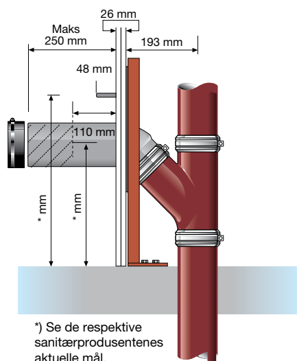
Fig. 2. Tilkobling av vegghengt klosett rett foran vertikal samleledning med grnør 45° og kappbart klosettend 45°.
