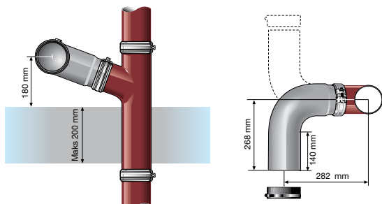
Fig. 1. Tilkobling av ett eller to klosetter med P-lås til side for vertikal samleledning med etasjegrnør 70° og enkelt eller dobbelt klosettend 90°.
